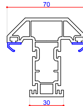
705549 (P10549) Chamf Comp Door T Transom Steel Box 713155 (S00155)
